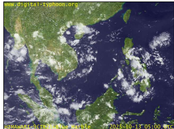
ภาพถ่ายดาวเทียม วันที่ ๑๓ ต.ค. ๒๕๖๘ เวลา ๑๒.๐๐ น.
